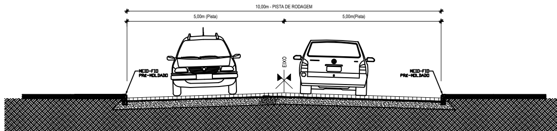
SEÇÃO TIPO DE BLOCO INTERTRAVADO - RUA GUAJUVIRA
